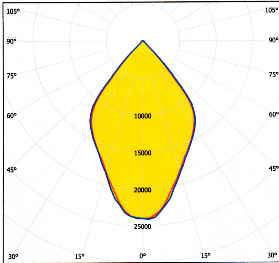
Рисунок 1 – КСС образца светильник светодиодный ET-CC-05-200 в поперечной (C0-C180) (красная кривая) и продольной (C90-C270) (синяя кривая) плоскостях
